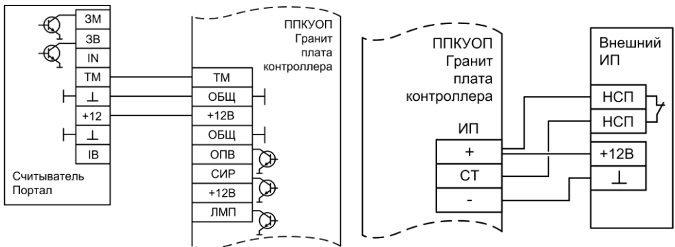
Рис.Б6 Схема подключения внешнего источника электропитания (ИП)
